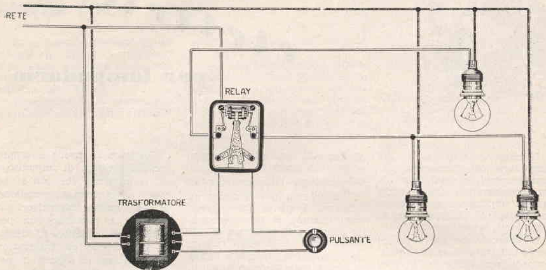
Fig. 2. — Impianto per lampadario con relay.
