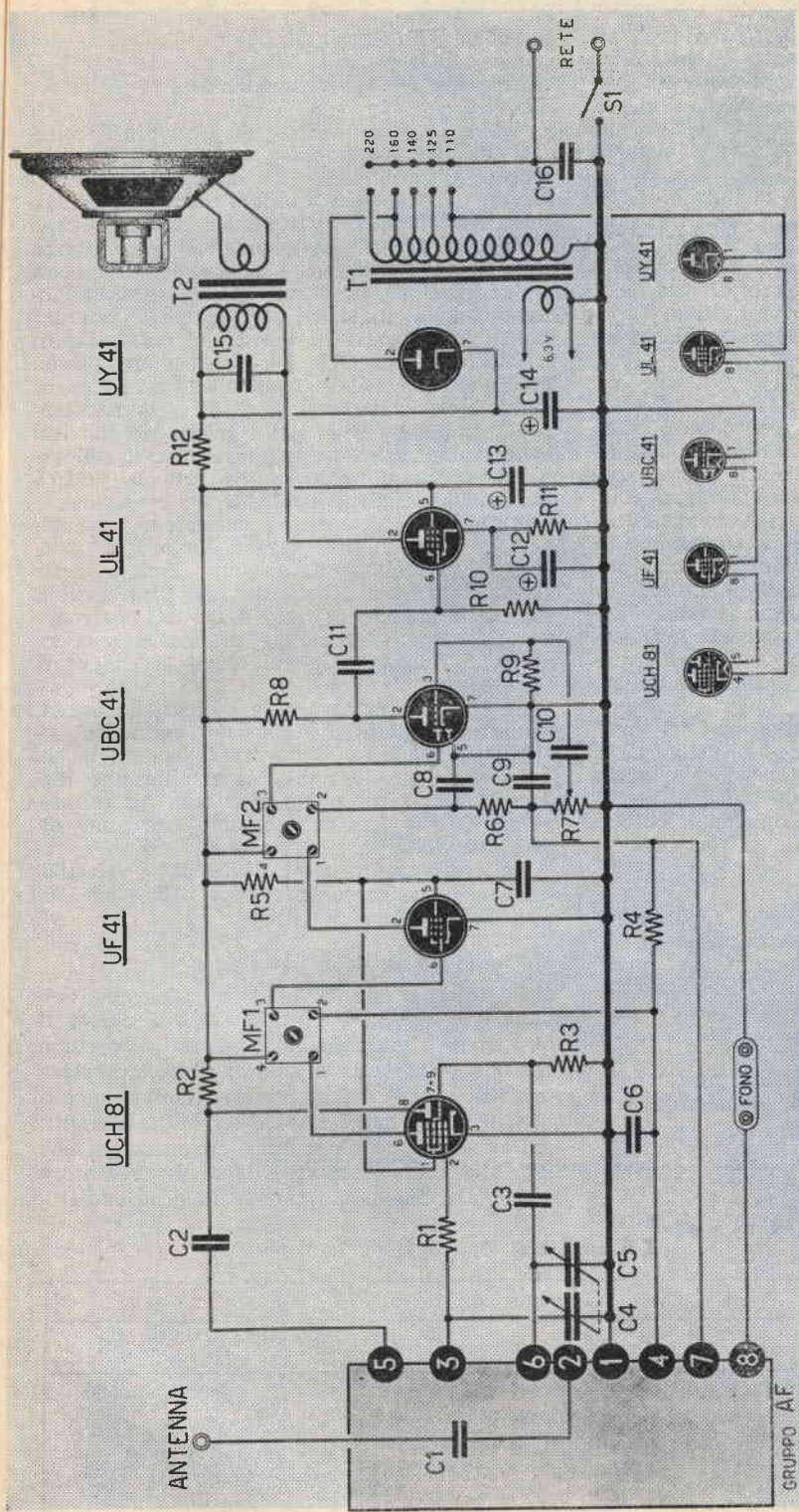
Fig. 1. — Schema elettrico.
