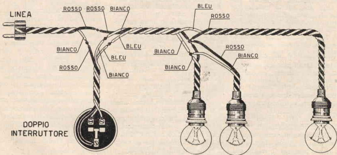
Fig. 1. — Impianto per lampadario con interruttore doppio.
